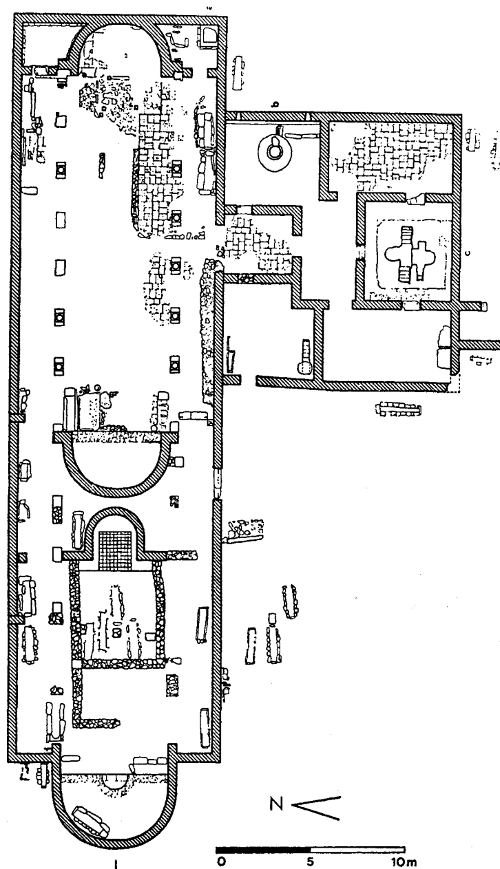
Planta de la iglesia de la villa de Torre de Palma, Monforte, Portugal, según Almeida-Martins de Martos.
