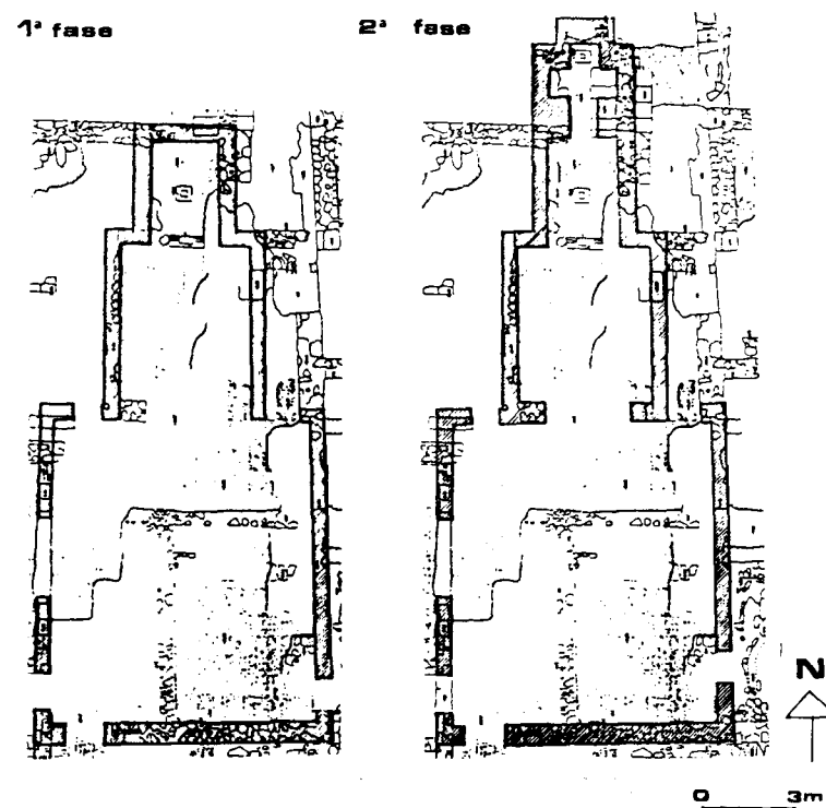
Planta de la basílica paleocristiana de Conímbriga (Lusitania), según M. Justino Maciel y T. Campos Coelho.
