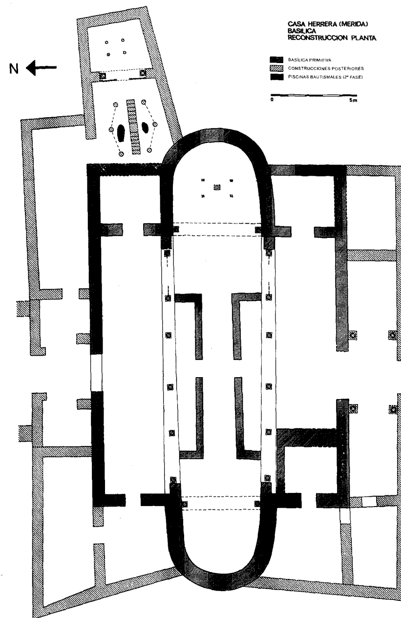
Distribución de los espacios litúrgicos en la iglesia de Casa Herrera, Mérida, según Caballero y Ulbert.
